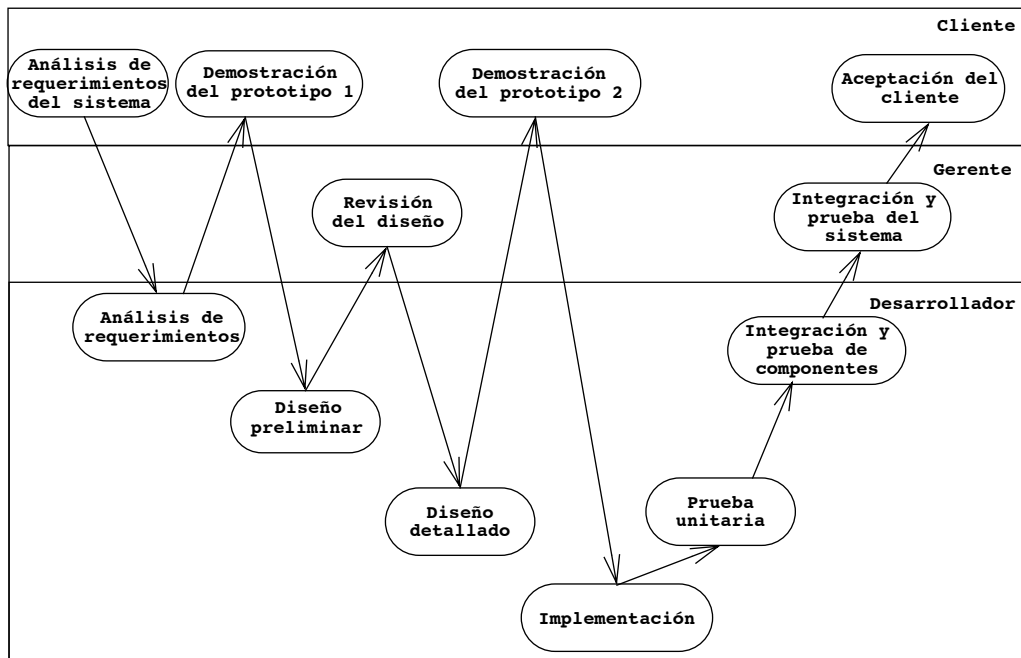
Figura 12-13 El modelo de diente de tiburón con dos demostraciones de prototipo y una revisión (diagrama de actividad UML, los niveles de abstracción están representados con carriles). Los dientes pequeños que llegan al carril del gerente son revisiones internas que involucran una demostración de prototipo hecha por los desarrolladores para el gerente del proyecto. Los dientes grandes que llegan al carril del cliente son demostraciones de prototipo para el cliente.
