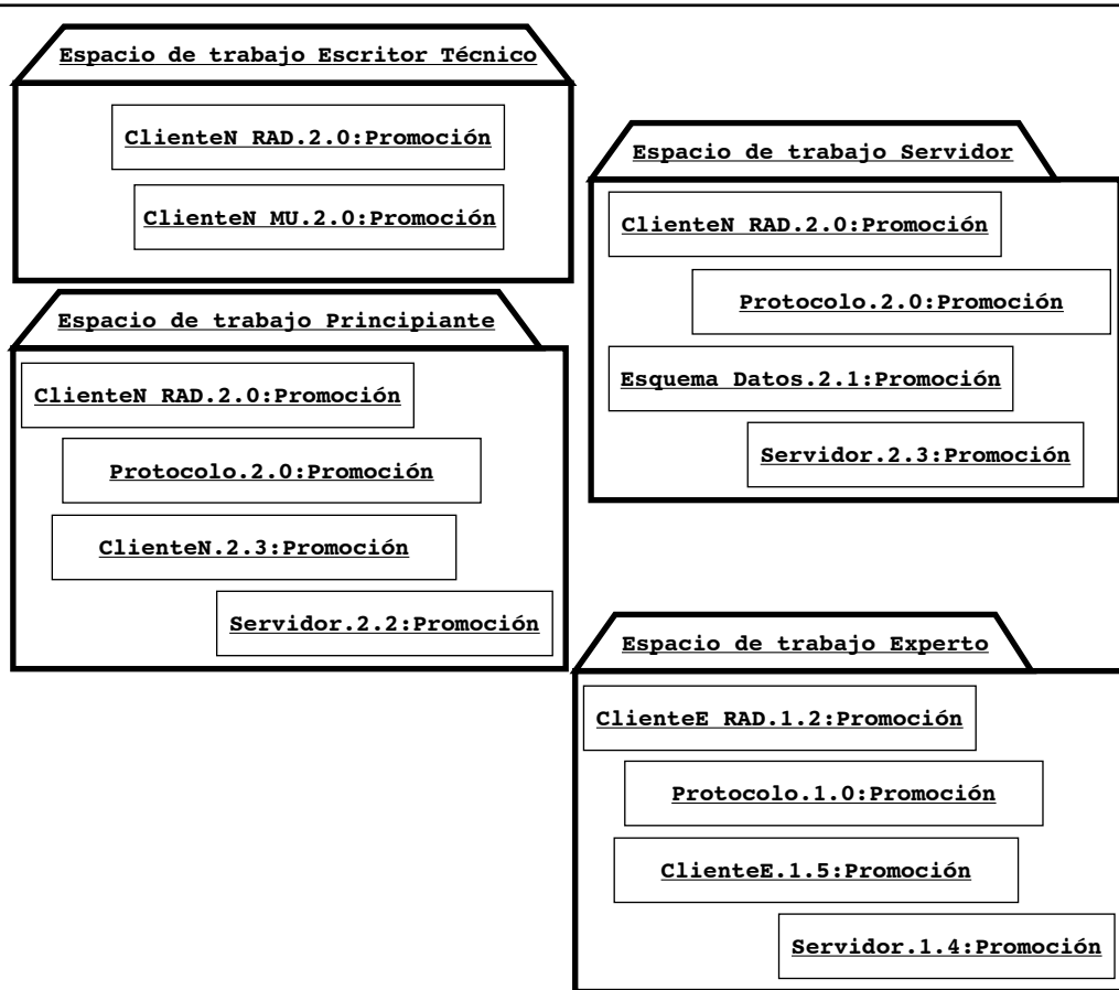
Figura 10-9 Instantánea de los espacios de trabajo usados por los desarrolladores de MisPartesCarro (diagrama de objetos UML). Los espacios de trabajo Principiante, Escritor Técnico y Servidor contienen promociones relacionadas con la funcionalidad del mapa de navegación. Sin embargo, el espacio de trabajo Experto contiene versiones antiguas y más estables. Para todos los artículos de configuración, los números de versión de la forma 1.x se refieren a las promociones sin la funcionalidad de mapas de navegación, mientras que los números de versión de la forma 2.x se refieren a las promociones que contienen implementaciones parciales o completas de los mapas de navegación.
