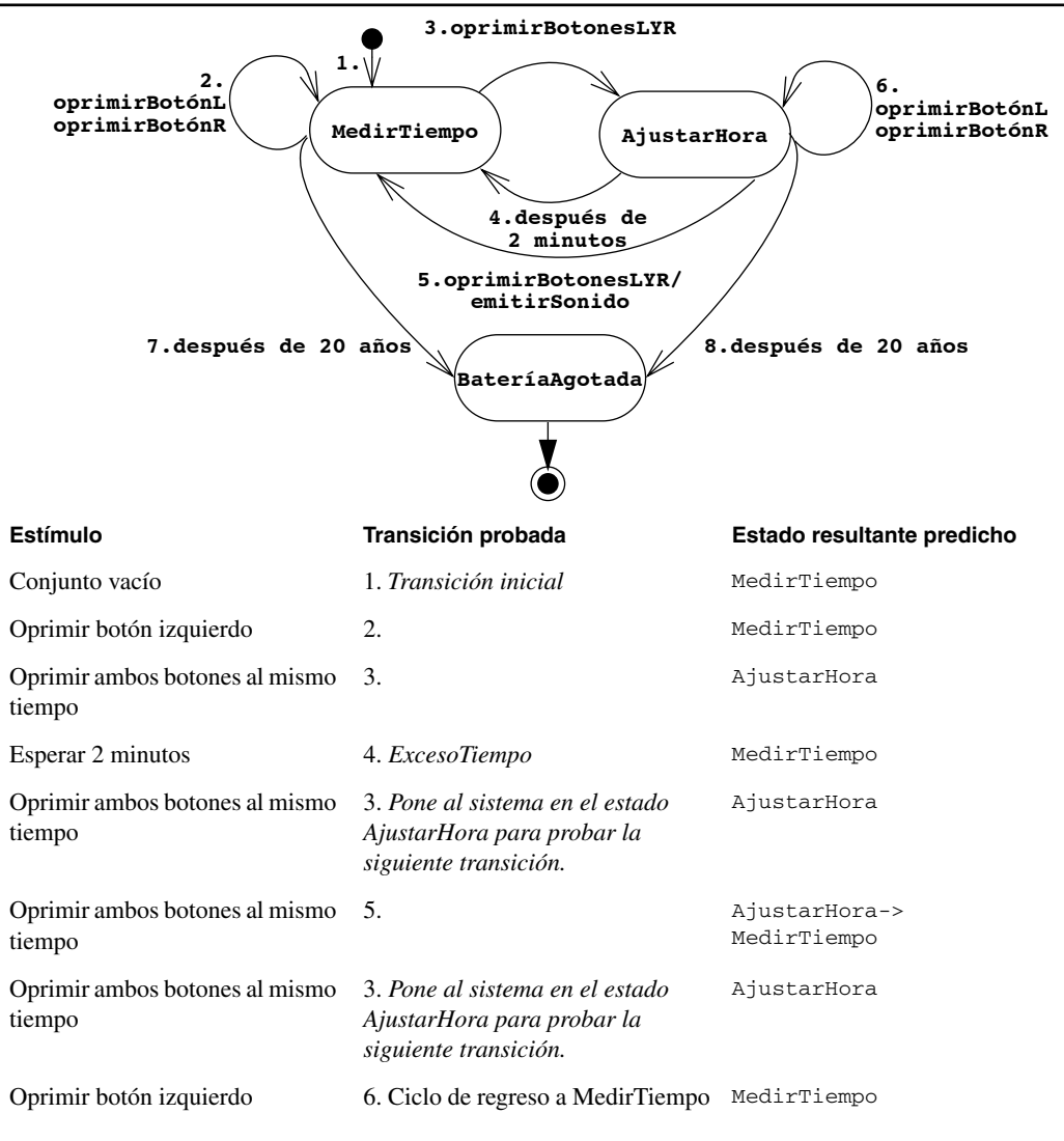
Figura 9-16 Diagrama de estado UML y pruebas resultantes para la función de ajustar la hora de Reloj2B. Sólo se muestran los primeros ocho estímulos.
