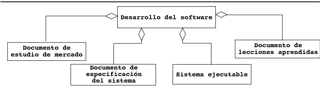
Figura 12-4 Visión centrada en entidad del desarrollo de software (diagrama de clase UML).
