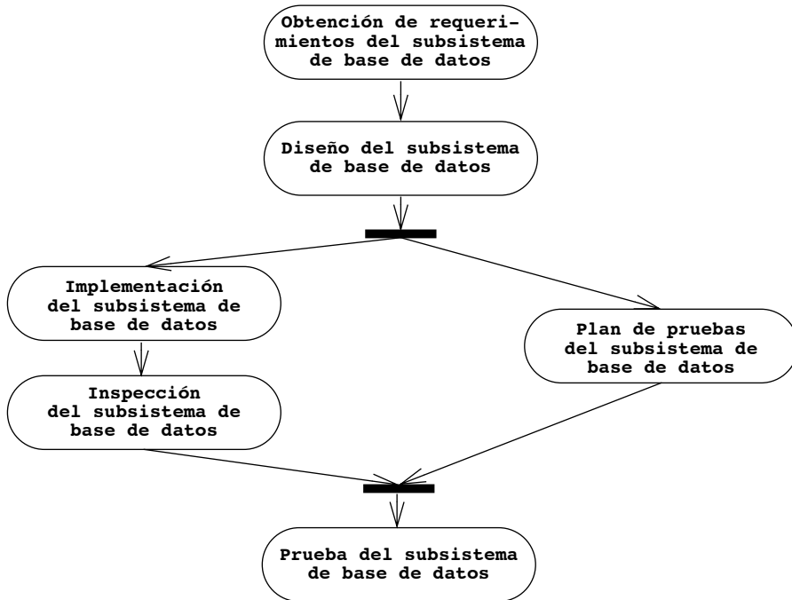
Figura 11-8 Un ejemplo de un modelo de tareas con dependencias de precedencia para el ejemplo de subsistema de base de datos de la tabla 11-1 (diagrama de actividad UML).
