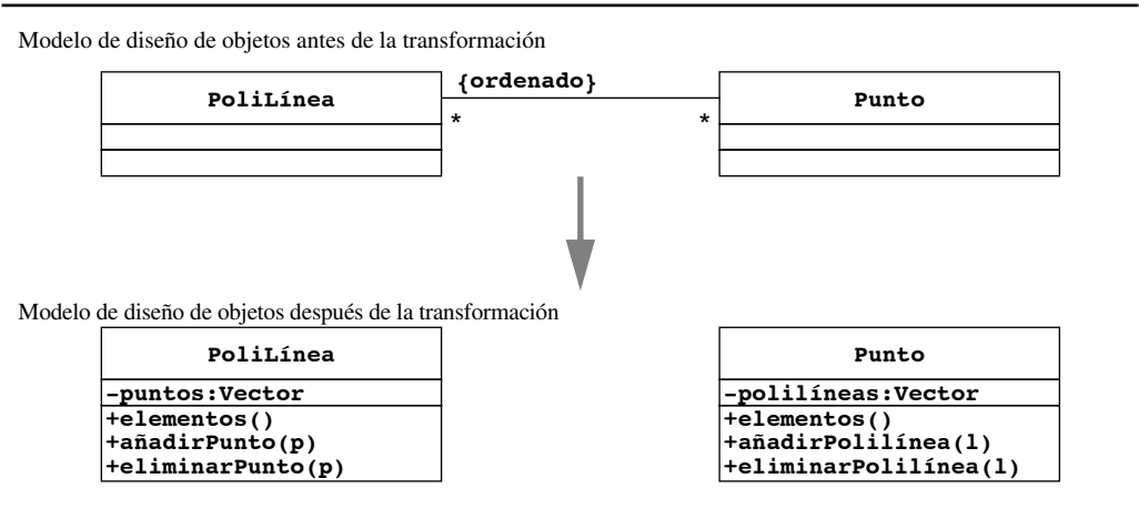
Figura 7-24 Realización de una asociación bidireccional de muchos a muchos (diagrama de clase UML; la flecha indica la transformación del modelo de diseño de objetos).
