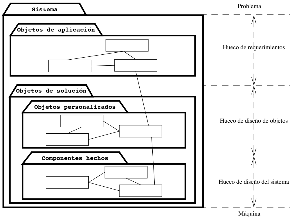
Figura 7-1 El diseño de objetos cierra el hueco entre los objetos de aplicación identificados durante los requerimientos y los componentes hechos seleccionados durante el diseño del sistema (diagrama de clase UML estilizado).
