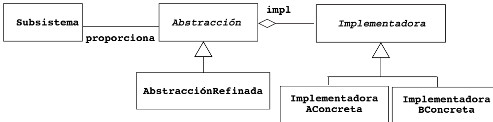
Figura 6-36 Patrón Puente (diagrama de clase UML).
