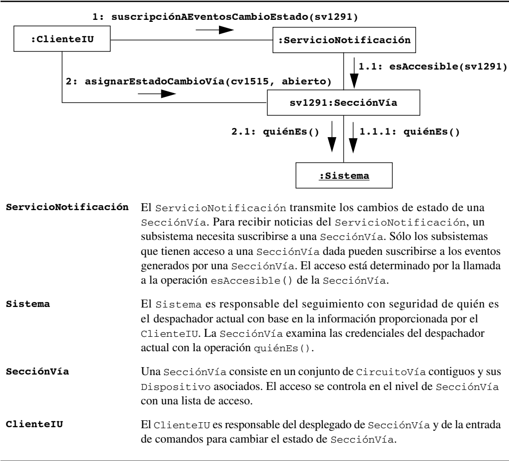
Figura 8-14 Propuesta P[1] : el acceso es controlado por el objeto SecciónVía con una lista de acceso. El ServicioNotificación consulta a la SecciónVía para determinar si un subsistema puede recibir noticias acerca de una SecciónVía dada (diagrama de colaboración UML).
