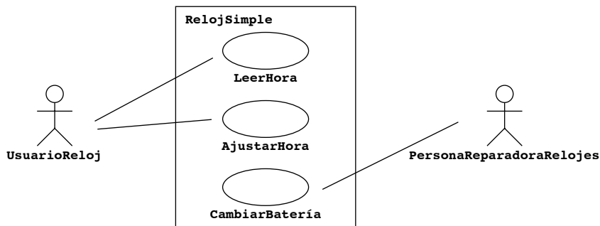
Figura 2-1 Un diagrama de caso de uso UML que describe la funcionalidad de un reloj simple. El actor UsuarioReloj puede consultar la hora en su reloj (con el caso de uso LeerHora ) o ajustar la hora (con el caso de uso AjustarHora ). Sin embargo, sólo el actor PersonaReparadoraReloj puede cambiar la batería del reloj (con el caso de uso CambiarBatería ). Los actores se representan con muñequitos (“hombres de paja”), los casos de uso con óvalos y la frontera del sistema con un cuadro que encierra los casos de uso.
