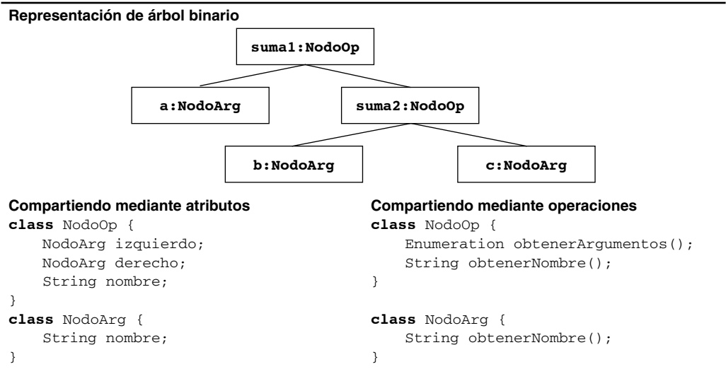
Figura 6-5 Ejemplo de una reducción de acoplamiento (diagrama de objetos UML y declaraciones Java). Esta figura muestra un árbol de análisis para la expresión “a + b + c”. La columna izquierda muestra la interfaz de la clase NodoOp compartiéndola mediante atributos. La columna derecha muestra la interfaz de NodoOp compartiéndola mediante operaciones. La figura 6-6 muestra los cambios para cada caso cuando, en vez de esto, se selecciona una lista vinculada.
