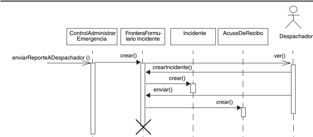
Figura 5-13 Diagrama de secuencia para el caso de uso ReportarEmergencia (EstaciónDespachador).
