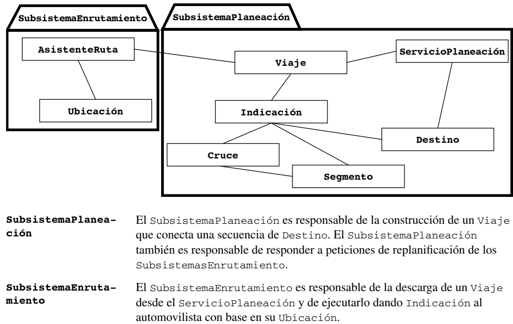
Figura 6-29 Descomposición en subsistemas inicial para MiViaje (diagrama de clase UML).
