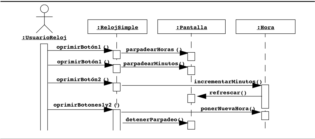
Figura 2-3 Un diagrama de secuencia UML para el RelojSimple. La columna de la extrema izquierda representa la línea de tiempo del actor UsuarioReloj, quien inicia el caso de uso. Las demás columnas representan la línea de tiempo de los objetos que participan en este caso de uso. Los nombres de objetos están subrayados para indicar que son instancias (en vez de clases). Las flechas etiquetadas son estímulos que envía un actor o un objeto a otros objetos.
