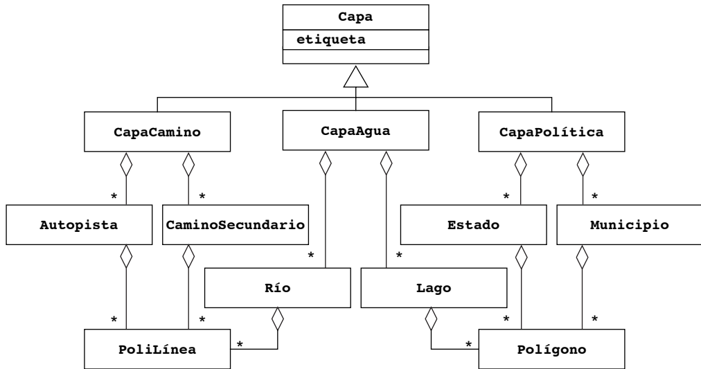
Figura 7-7 Modelo de objetos para el GIS de JEWEL (diagrama de clase UML).
