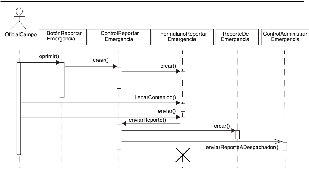
Figura 5-12 Diagrama de secuencia para el caso de uso ReportarEmergencia (inicio desde el lado de EstaciónOficialCampo).
