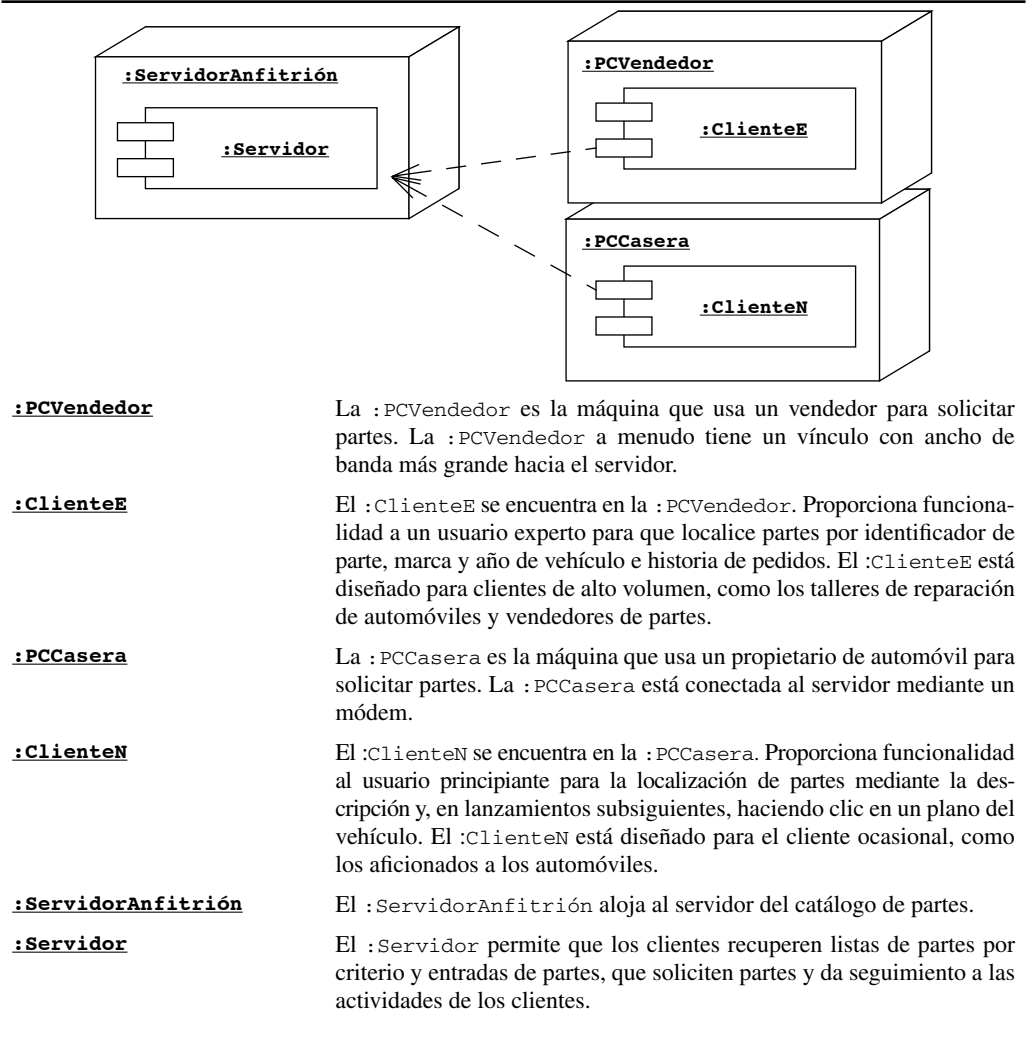
Figura 10-7 Descomposición en subsistemas de MisPartesCarro y asignación de hardware (diagrama de distribución UML).
