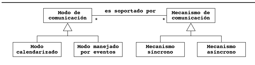
Figura 3-1 Clasificación de los modos y mecanismos de comunicación (diagrama de clase UML).
