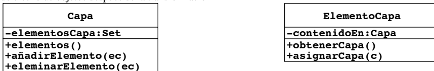
Figura 7-23 Realización de una asociación bidireccional de uno a muchos (diagrama de clase UML; la flecha indica la transformación del modelo de diseño de objetos).
