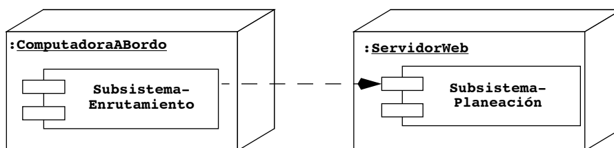
Figura 6-31 Asignación de los subsistemas de MiViaje al hardware (diagrama de organización UML). SubsistemaEnrutamiento ejecuta en :ComputadoraABordo y SubsistemaPlaneación ejecuta en :ServidorWeb .
