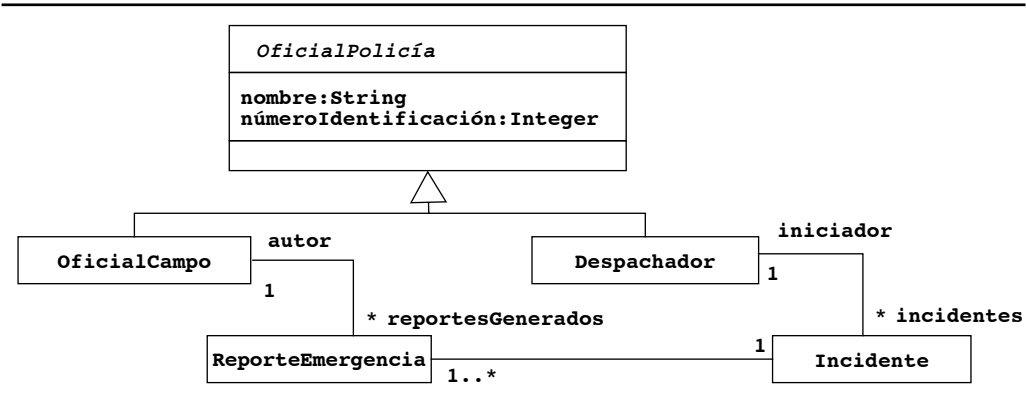
Figura 2-27 Un ejemplo de generalización (diagrama de clase UML). OficialPolicía es una clase abstracta que define los atributos y operaciones comunes de las clases OficialCampo y Despachador .
