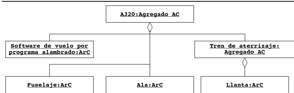
Figura 10-2 Un ejemplo de agregados AC y artículos de configuración (diagrama de objetos UML).
