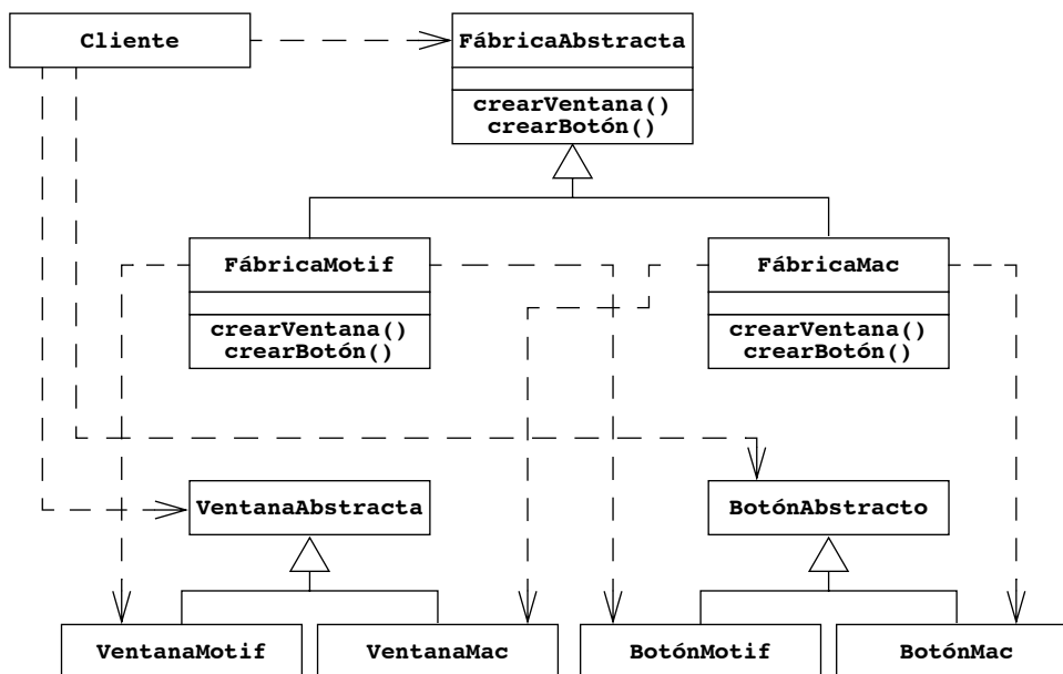
Figura 7-28 Patrón de diseño FábricaAbstracta (diagrama de clase UML, las dependencias representan relaciones <<llama>> ). Este patrón de diseño usa herencia para soportar diferentes apariencias (por ejemplo, Motif y Macintosh). Si se añade una nueva especialización no es necesario cambiar al cliente.
