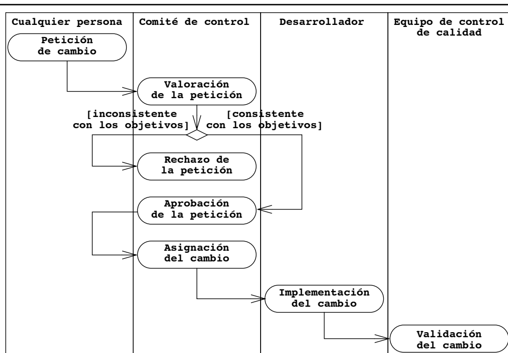
Figura 10-14 Un ejemplo del proceso de administración del cambio (diagrama de actividad UML).
