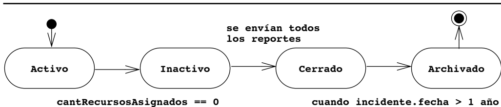
Figura 5-19 Gráfica de estado UML para Incidente .
