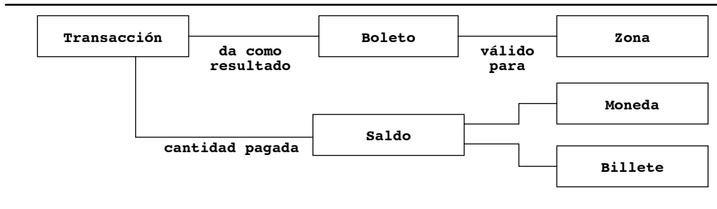
Figura 1-3 Un modelo de objeto para el distribuidor de boletos (diagrama de clase UML). En el caso de uso CompraBoletoSencillo , un Viajero inicia una transacción que dará como resultado un Boleto . Un Boleto es válido solo para una Zona especificada. Durante la Transacción , el sistema calcula el Saldo contando las Monedas y Billetes insertados.
