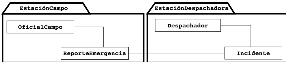
Figura 2-41 Ejemplo de paquetes. Las clases OficialCampo y ReporteEmergencia se encuentran en el paquete EstaciónCampo , y las clases Despachador e Incidente se encuentran en el paquete EstaciónDespachadora .
