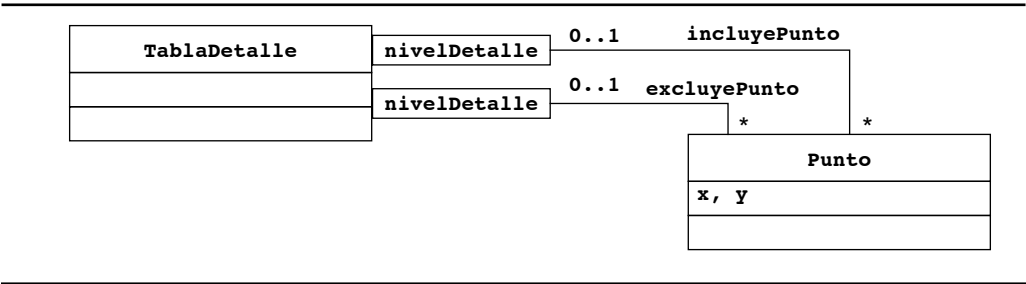
Figura 7-34 TablaDetalle es un objeto global que lleva cuenta de cuáles Punto han sido incluidos o excluidos de un nivelDetalle especificado. Ésta es una alternativa para los conjuntos enNivelesDetalle y noEnNivelesDetalle que se muestran en la figura 7-14.
