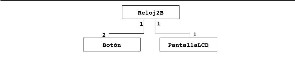
Figura 5-5 Un ejemplo de multiplicidad de asociaciones (diagrama de clase UML). Un Reloj2B tiene dos botones y una PantallaLCD.
