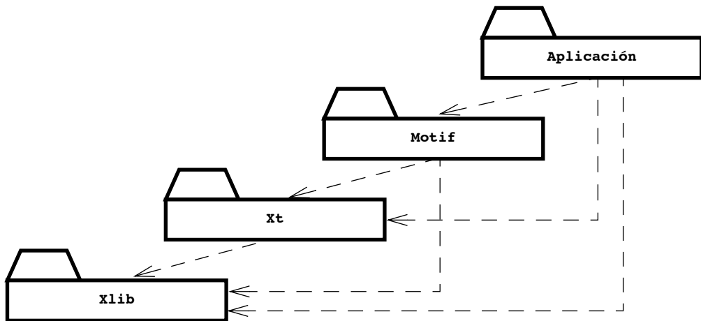
Figura 6-12 Un ejemplo de arquitectura abierta: la biblioteca OSF/Motif (diagrama de clase UML, paquetes colapsados). Xlib proporciona facilidades de trazado de bajo nivel. Xt proporciona el manejo de aparatos mecánicos de interfaz de usuario básicos. Motif proporciona una gran cantidad de aparatos mecánicos sofisticados. La Aplicación puede tener acceso a cada una de estas capas en forma independiente.
