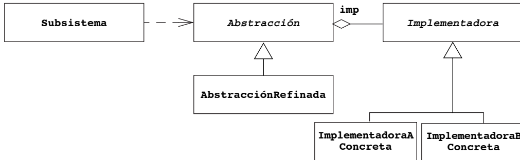
Figura A-3 Patrón Puente (diagrama de clase UML).
