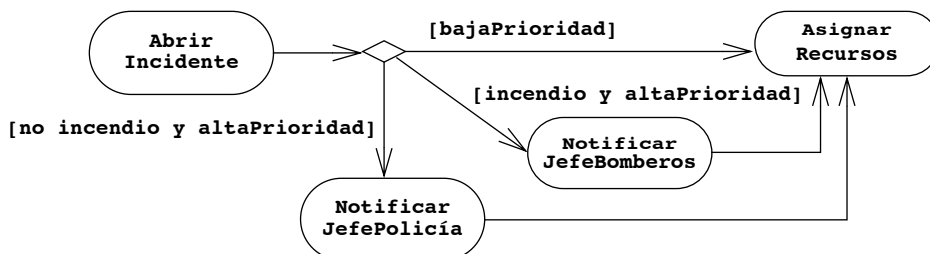
Figura 2-36 Ejemplo de decisiones en el proceso Abrir Incidente . Si el Incidente es un incendio y es de alta prioridad, el Despachador le notifica al JefeBomberos . Si el incidente es de alta prioridad y no es un incendio, se notifica al JefePolicía . En todos los casos, el Despachador asigna recursos para manejar el Incidente.
