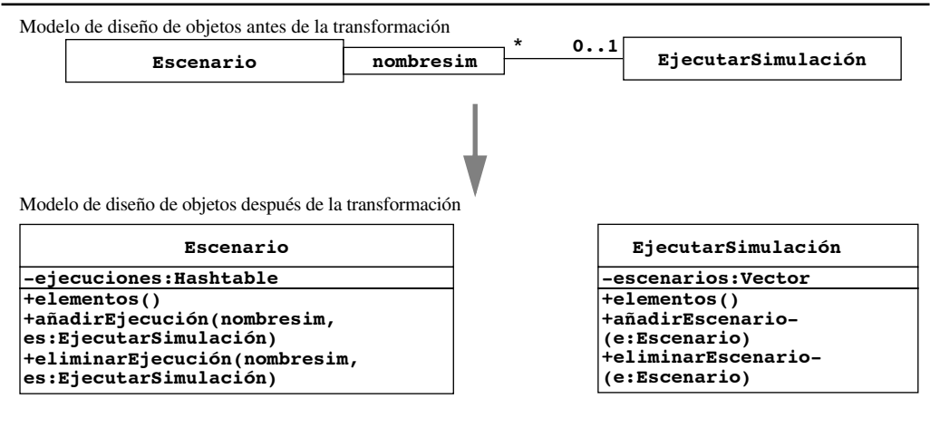
Figura 7-26 Realización de una asociación bidireccional calificada (diagrama de clase UML; la flecha indica la transformación del modelo de diseño de objetos).
