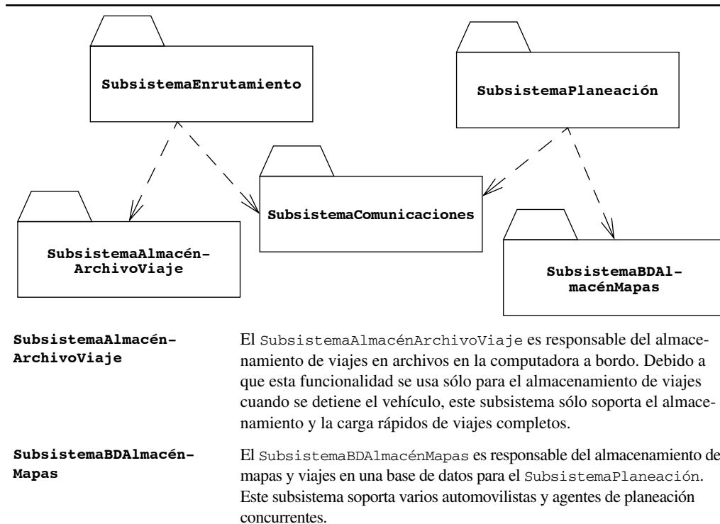
Figura 6-35 Descomposición en subsistemas de MiViaje después de decidir sobre los asuntos de almacenamiento de datos (diagrama de clase UML, paquetes colapsados por claridad).
