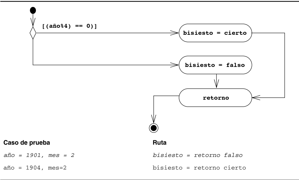
Figura 9-15 Diagrama de flujo equivalente para la implementación (defectuosa) del método esAño-Bisiesto() de la figura 9-14 (diagrama de actividad UML) y pruebas derivadas. La prueba en cursivas es redundante con una prueba que derivamos del método obtenerNumDíasEnMes() .
