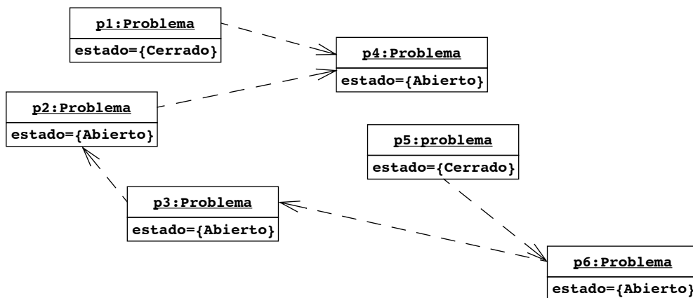
Figura 12-15 Instantánea de una base de problemas de proyecto (diagrama de objetos UML). Los problemas p_1 y p_5 ya se han resuelto, mientras que todos los demás todavía están abiertos. Las dependencias entre problemas indican que la resolución de un problema puede restringir las alternativas para los problemas dependientes.
