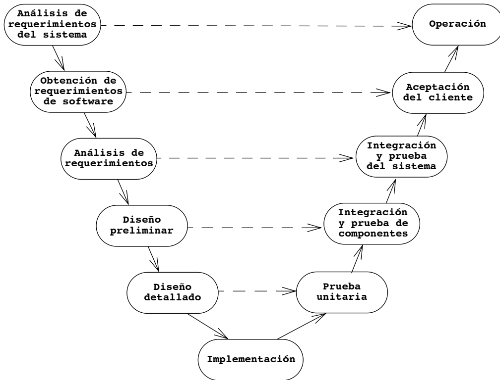
Figura 12-10 Modelo V de desarrollo de software (diagrama de actividad UML, adaptado de [Jensen y Tonies, 1979]). El flujo de objetos horizontal indica el flujo de información entre las actividades del mismo nivel de abstracción (por ejemplo, los resultados del análisis de requerimientos del sistema se validan durante la integración y prueba del sistema). Se conservó la disposición de las actividades en forma de V para reflejar el trazo original. Sin embargo, la disposición de las actividades no tiene semántica en UML.
