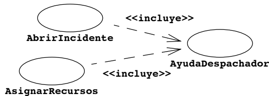
Figura 2-18 Un ejemplo de una relación <<incluye>> (diagrama de caso de uso UML).
