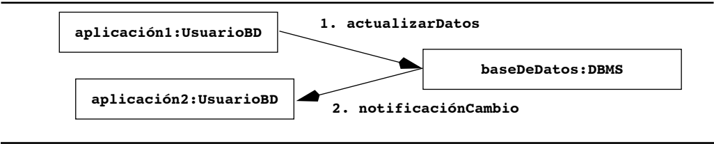
Figura 6-21 Un ejemplo de arquitectura par a par (diagrama de colaboración UML). El servidor de base de datos puede procesar peticiones de las aplicaciones y enviar notificaciones a éstas.
