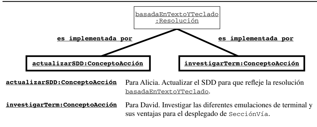
Figura 8-8 Un ejemplo de implementación de una resolución (diagrama de objetos UML). Los ConceptoAcción se resaltan en negritas.
