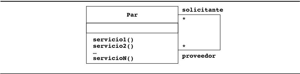
Figura 6-20 Arquitectura par a par (diagrama de clase UML). Los pares pueden solicitar y proporcionar servicios a los demás pares.
