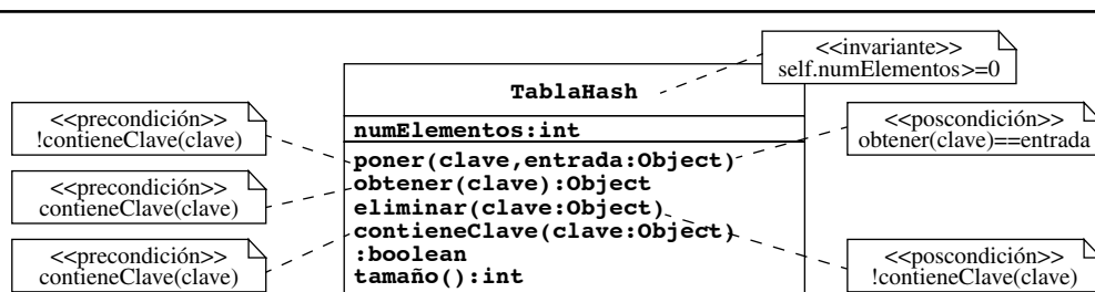
Figura 7-5 Ejemplos de invariantes, precondiciones y poscondiciones en OCL (diagrama de clase UML).
