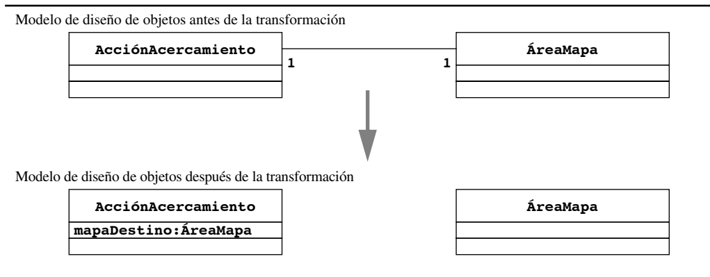
Figura 7-21 Realización de una asociación unidireccional de uno a uno (diagrama de clase UML; la flecha indica la transformación del modelo de objetos).
