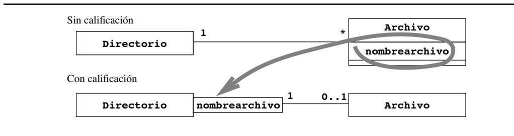
Figura 5-9 Ejemplo de la manera en que la asociación calificada reduce la multiplicidad (diagrama de clase UML). La adición de un calificador aclara el diagrama de clase e incrementa la información que conlleva. En este caso, el modelo que incluye la calificación indica que el nombre del archivo es único dentro de un directorio.
