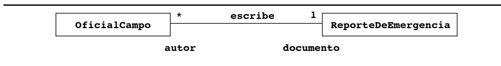
Figura 5-16 Un ejemplo de asociación entre las clases ReporteDeEmergencia y OficialCampo .
