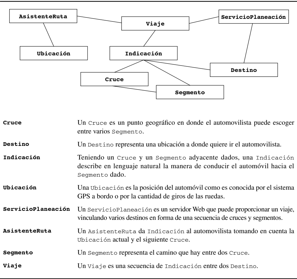
Figura 6-28 Modelo de análisis para la planeación y ejecución de la planeación de ruta de MiViaje.
