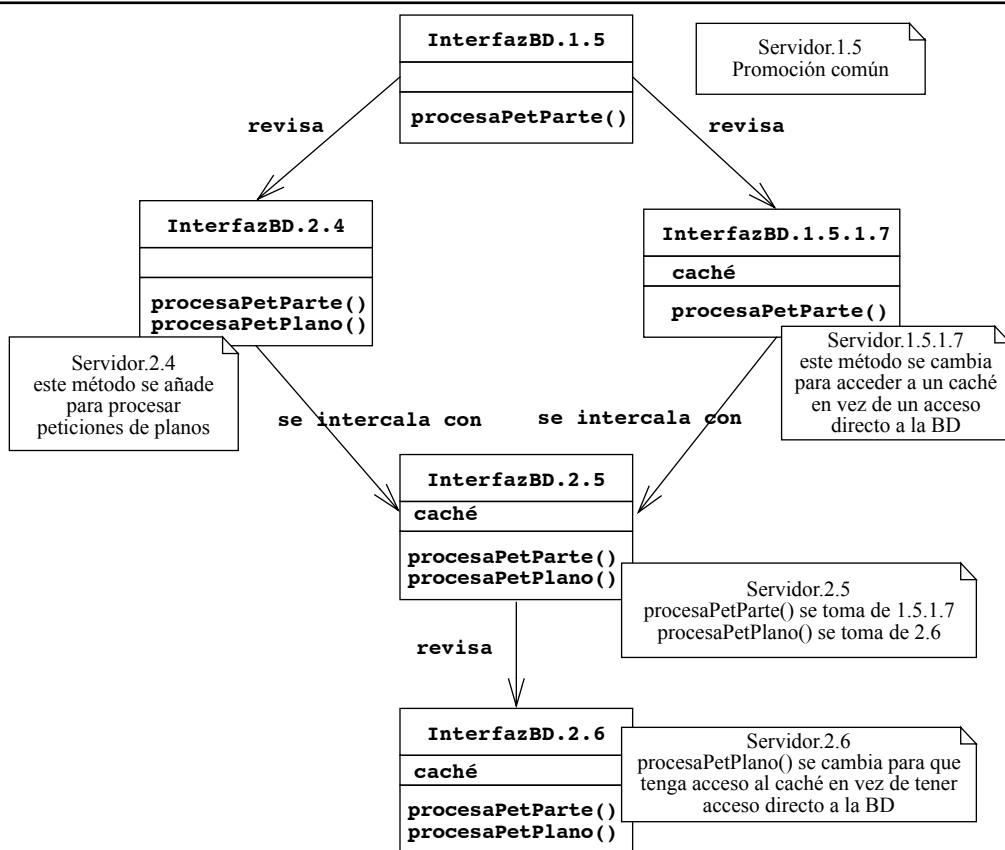
Figura 10-12 Un ejemplo de una intercalación de la clase InterfazBD del sistema MisPartesCarro (diagrama de clase UML).
