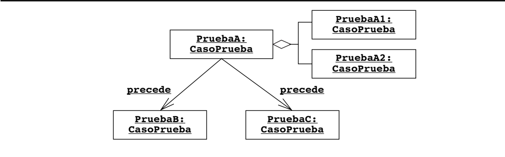
Figura 9-10 Modelo de prueba con casos de prueba. La PruebaA consiste en dos pruebas, PruebaA1 y PruebaA2. PruebaB y PruebaC pueden probarse de manera independiente, pero sólo después de que se haya realizado PruebaA.
