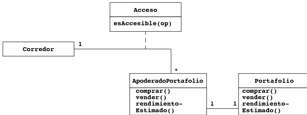
Figura 6-38 El acceso dinámico implementado con un Apoderado de protección. La clase de asociación Acceso contiene un conjunto de operaciones que puede usar Corredor para tener acceso a un Portafolio. Cada operación de ApoderadoPortafolio revisa primero con la operación esAccesible() si el Corredor que llama tiene acceso legítimo. Una vez que se ha otorgado el acceso, ApoderadoPortafolio delega la operación al objeto Portafolio actual. Una asociación Acceso puede usarse para controlar el acceso a muchos Portafolio.
