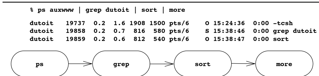
Figura 6-23 Una instancia de la arquitectura de tubo y filtro (comandos Unix y diagrama de actividad UML).
