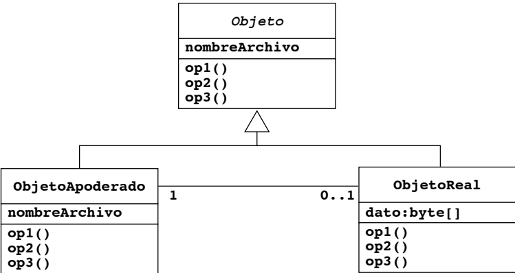
Figura A-8 El patrón Apoderado (Diagrama de clase UML).
