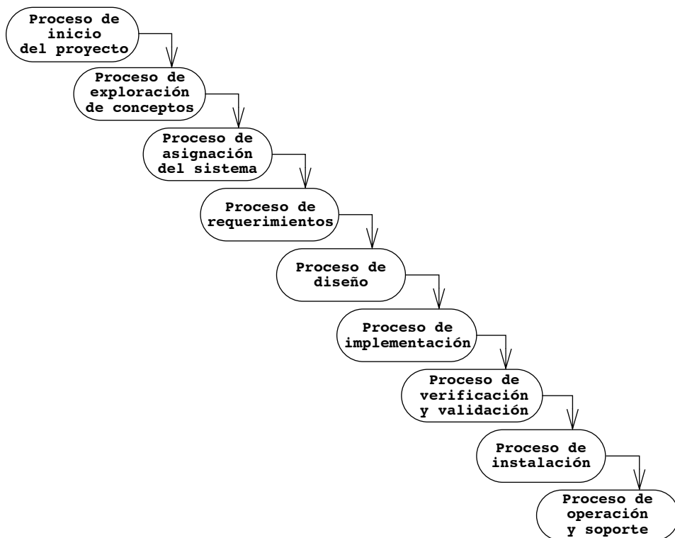
Figura 12-8 El modelo de cascada del desarrollo de software es una perspectiva centrada en actividad del ciclo de vida del software. Las actividades de desarrollo de software se realizan en secuencia (diagrama de actividad UML adaptado de [Royse, 1970] usando los nombres del IEEE 1074; se omiten los procesos de administración del proyecto y de desarrollo cruzado).
