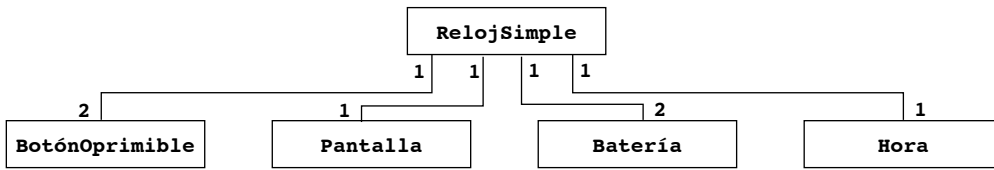
Figura 2-2 Un diagrama de clase UML que describe los elementos de un reloj simple.
