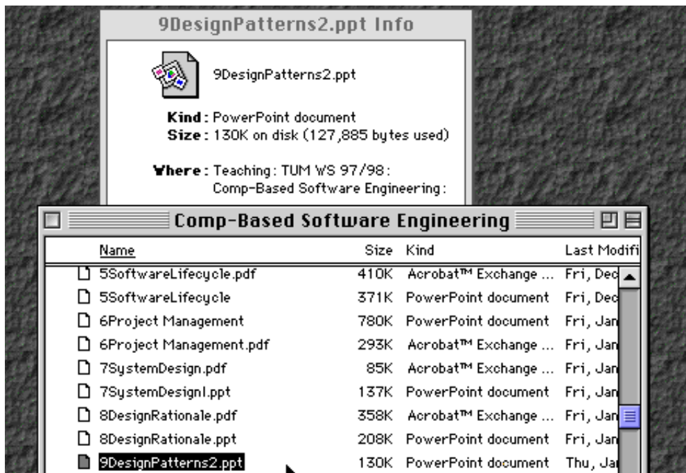
Figura 6-17 Un ejemplo de arquitectura MVC. El “modelo” es el nombre de archivo 9DesignPatterns2.ppt. Una “vista” es una ventana titulada Comp-Based Software Engineering que despliega el contenido de una carpeta que contiene el archivo 9DesignPatterns2.ppt. La otra “vista” es una ventana llamada 9DesignPatterns2.ppt Info que despliega información relacionada con el archivo. Si se cambia el nombre del archivo ambas vistas son actualizadas por el “controlador”.
