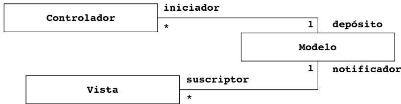
Figura 6-15 Arquitectura Modelo/Vista/Controlador (diagrama de clase UML). El Controlador recopila la entrada de los usuarios y envía mensajes al Modelo . El Modelo mantiene la estructura de datos central. La Vista despliega el Modelo y es notificada (mediante un protocolo de suscripción/notificación) cuando éste cambia.
