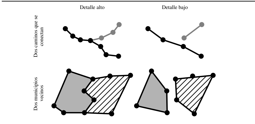
Figura 7-13 Un algoritmo de selección de puntos sencillo para el GIS. La columna izquierda representa un cruce de caminos y dos municipios vecinos. La columna derecha muestra que el cruce de caminos y los municipios vecinos pueden mostrarse en forma incorrecta cuando no se tiene cuidado en la selección de puntos.
