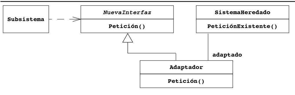
Figura A-2 Patrón Adaptador (diagrama de clase UML). El patrón Adaptador se usa para proporcionar una interfaz diferente ( NuevaInterfaz ) a un componente existente ( SistemaHeredado ).
