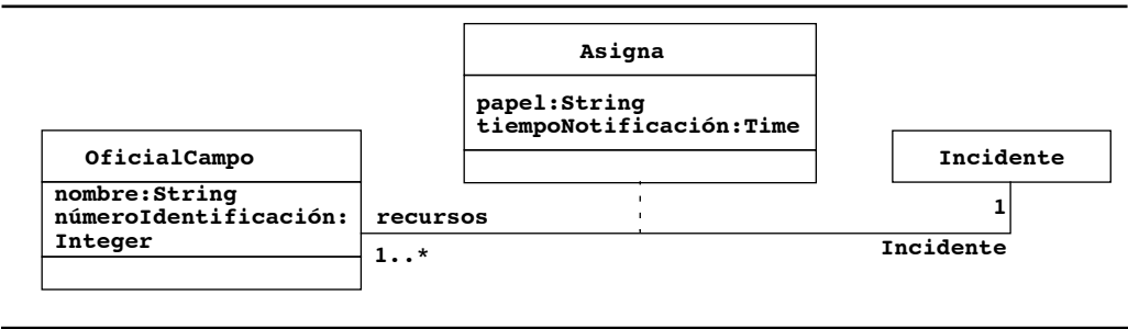
Figura 2-24 Un ejemplo de una clase de asociación (diagrama de clase UML).
