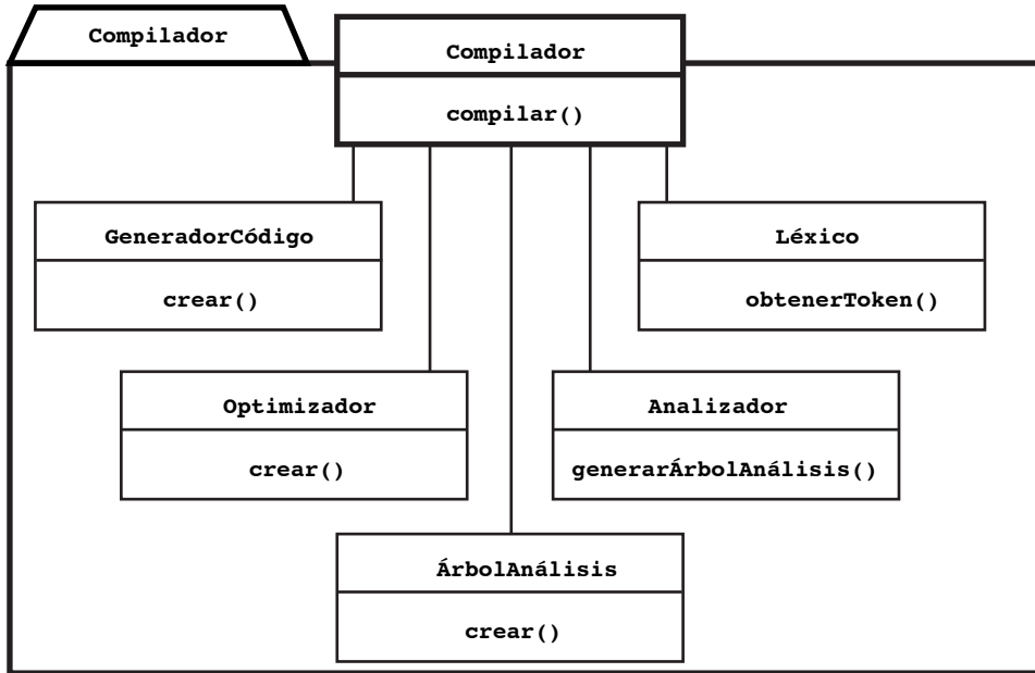
Figura A-6 Un ejemplo de un patrón Fachada (diagrama de clase UML).
