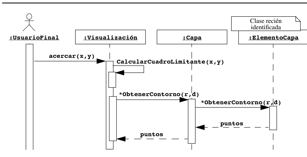
Figura 7-11 Un diagrama de secuencia para la operación acercar() (diagrama de secuencia UML). Este diagrama de secuencia conduce a la identificación de una nueva clase, ElementoCapa . Debido a que nos estamos enfocando en el GIS, tratamos al subsistema Visualización como un solo objeto.
