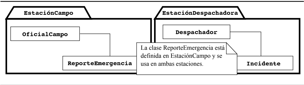
Figura 2-42 Un ejemplo de una nota. Se pueden añadir notas a un elemento específico de un diagrama.
