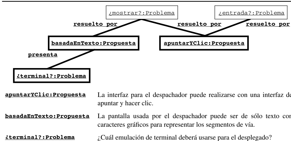
Figura 8-4 Un ejemplo de propuestas y problema consecuente (diagrama de objetos UML). Las Propuesta y el Problema consecuente se resaltan en negritas.
