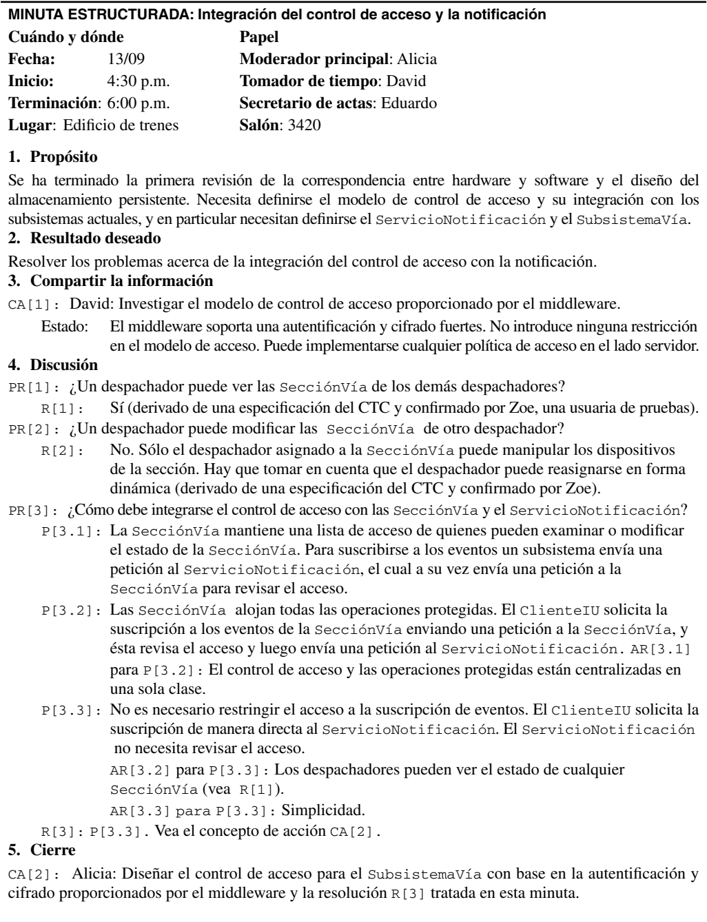
Figura 8-18 Minutas estructuradas de la discusión de control de acceso de CTC.
